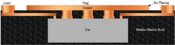
MDQFN
