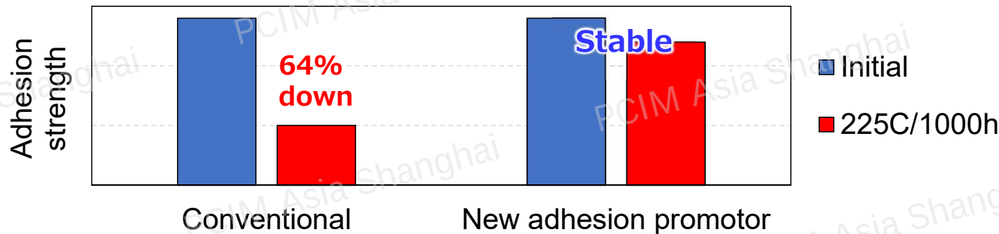
Cu adhesion @ 260degC
